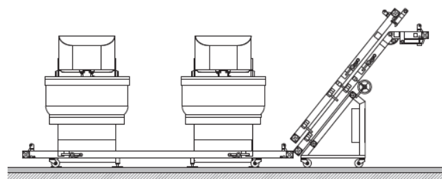
Konfigurationsexempel – två MD blandare med transportband under.
